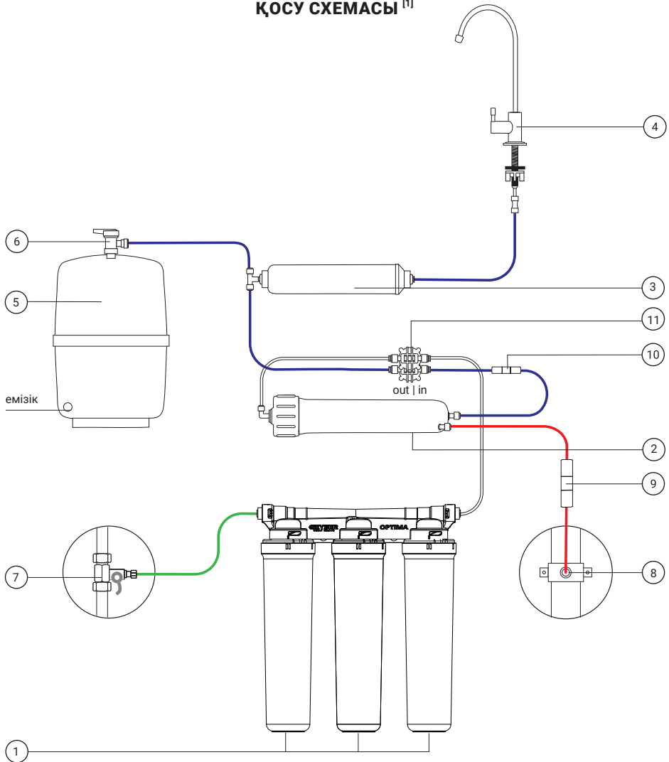
2-сур. Гейзер Престиж/Аллегро Оптимаы қосу схемасы.
